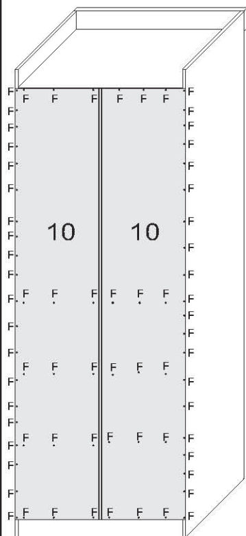
Móvel Vista Traseira
